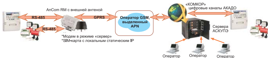
Рис. 9. Работа GSM-модемов в режиме минимизации трафика
