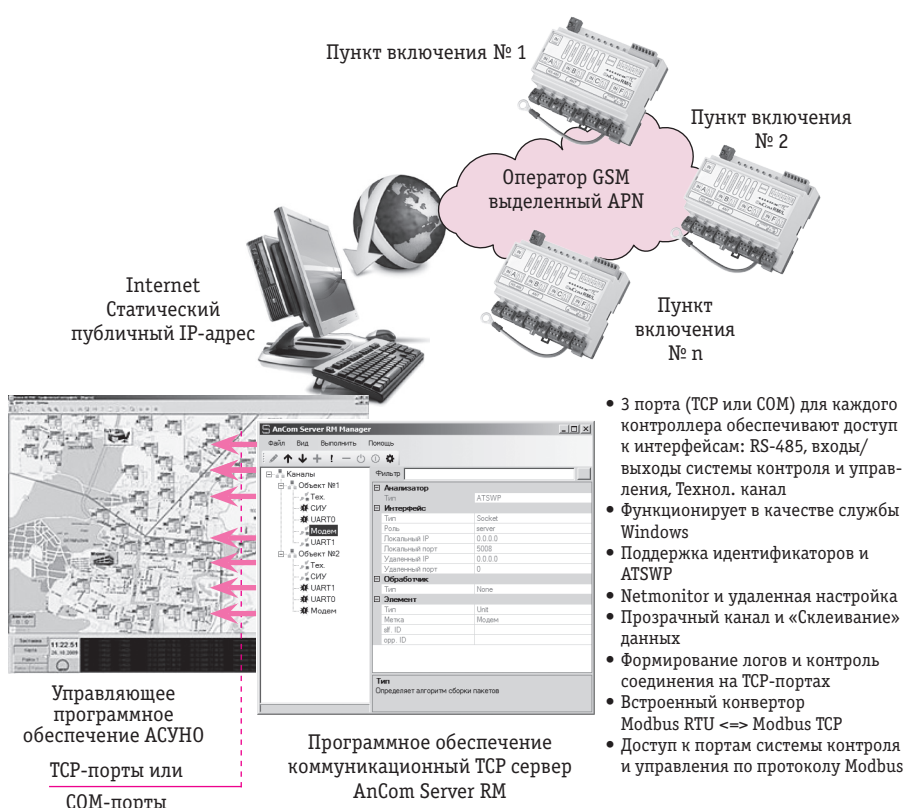
Рис. 4. Диспетчерский пункт
