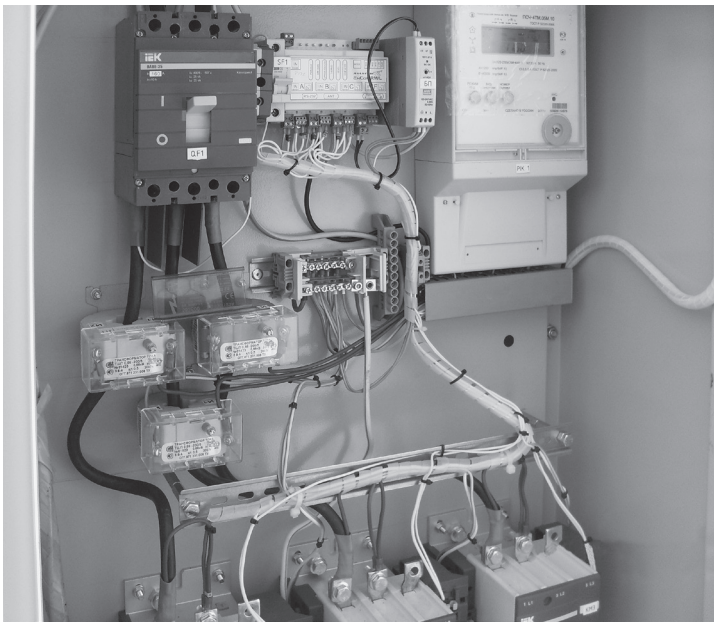
Рис. 6. Контроллер AnCom RM/L в составе пункта включения АСУНО на железнодорожной станции
