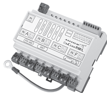
Рис. 1. Контроллер АСУНО AnCom RM/L RS-485, реле управления электромагнитными пускателями, входы контроля фазных напряжений и охранно-пожарной сигнализации, встроенный GPRS/EDGE модем
