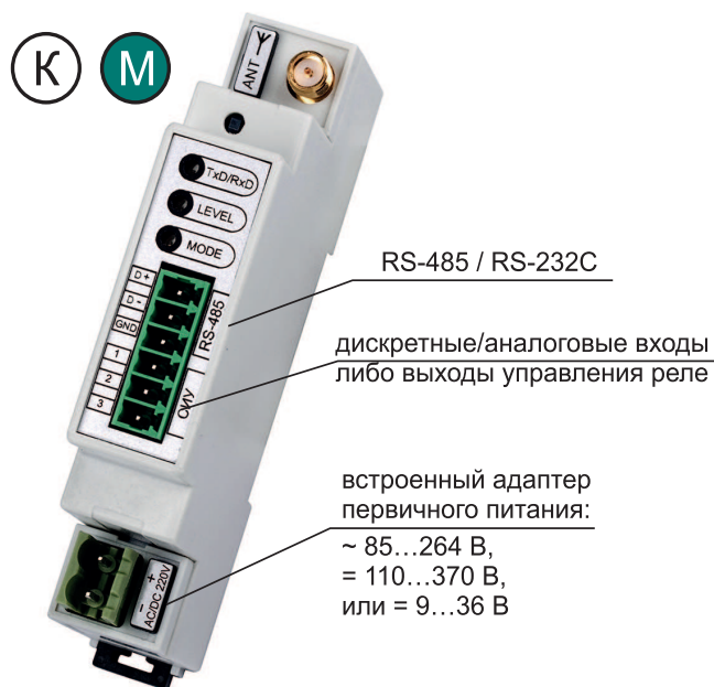
Рис. 1. ZigBee Pro модем AnCom RZ/B: крепление на DIN рейку, диапазон температур -40...70°С
