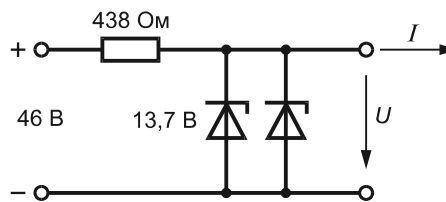
Рисунок С.3b — Эквивалентная цепь
