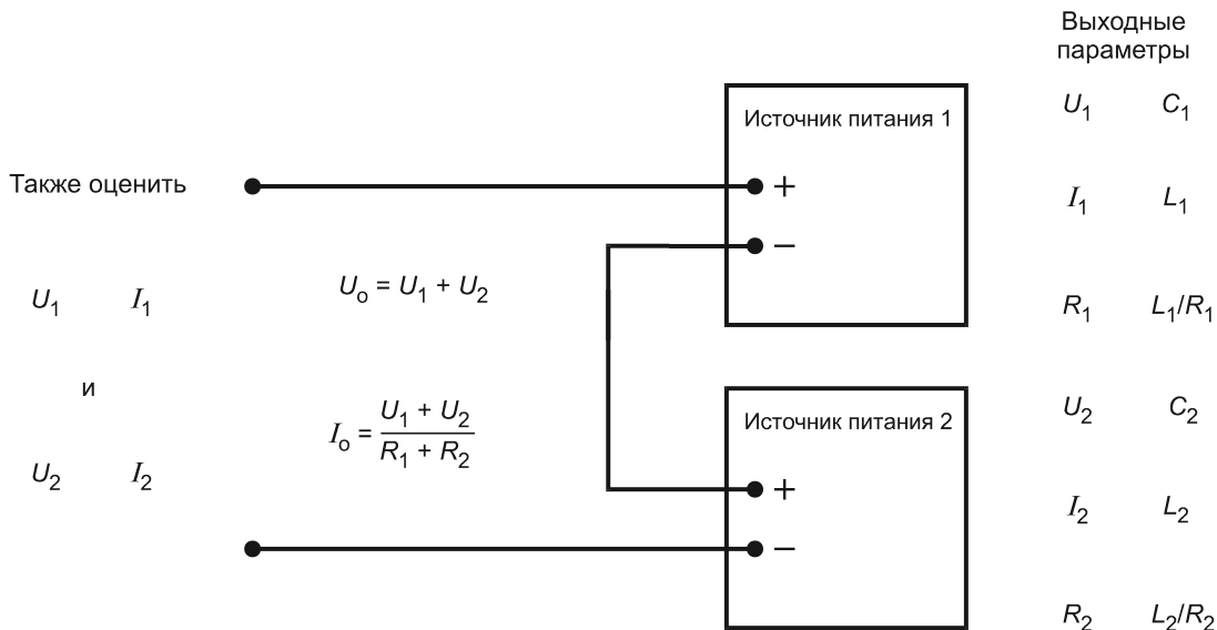
Рисунок В.1 — Источники питания, подключенные последовательно
