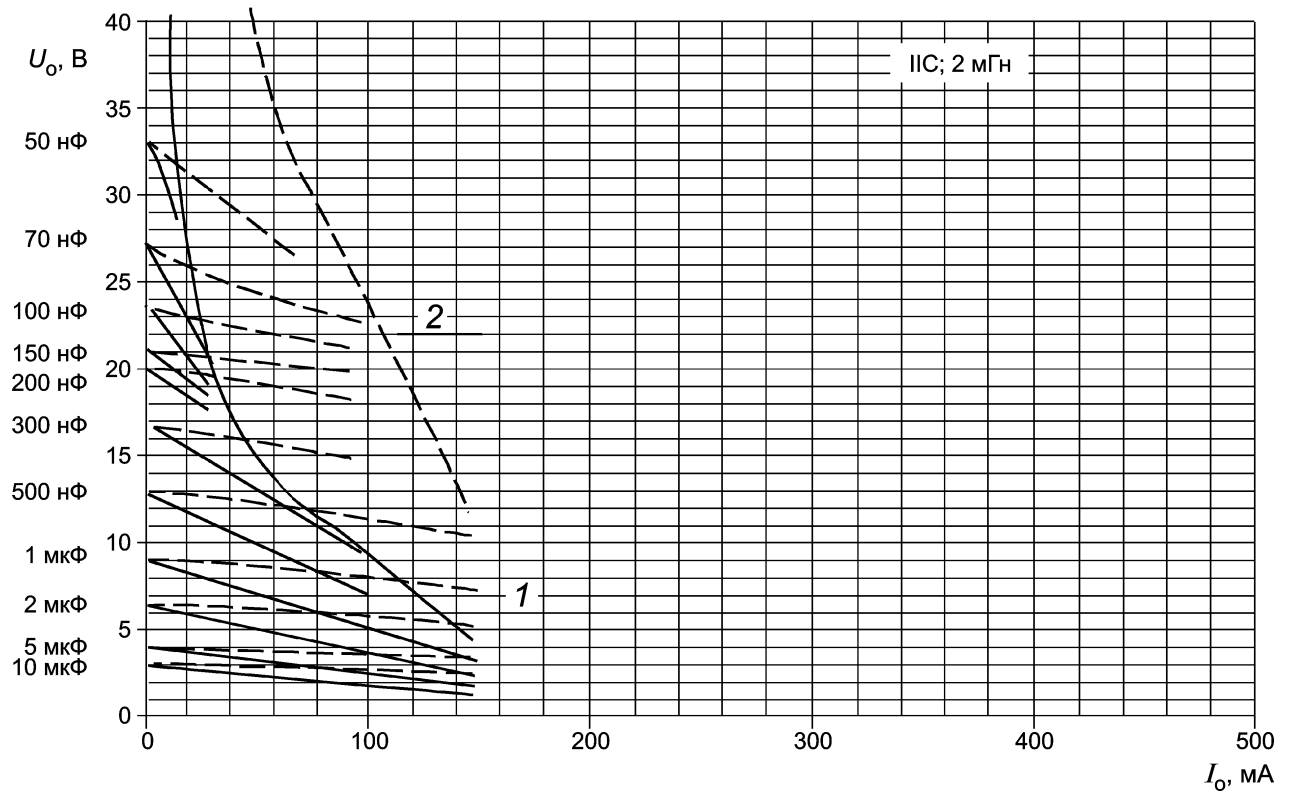
1 — максимальная индуктивность для источника с прямоугольной характеристикой; 2 — максимальная индуктивность для источника с линейной характеристикой
