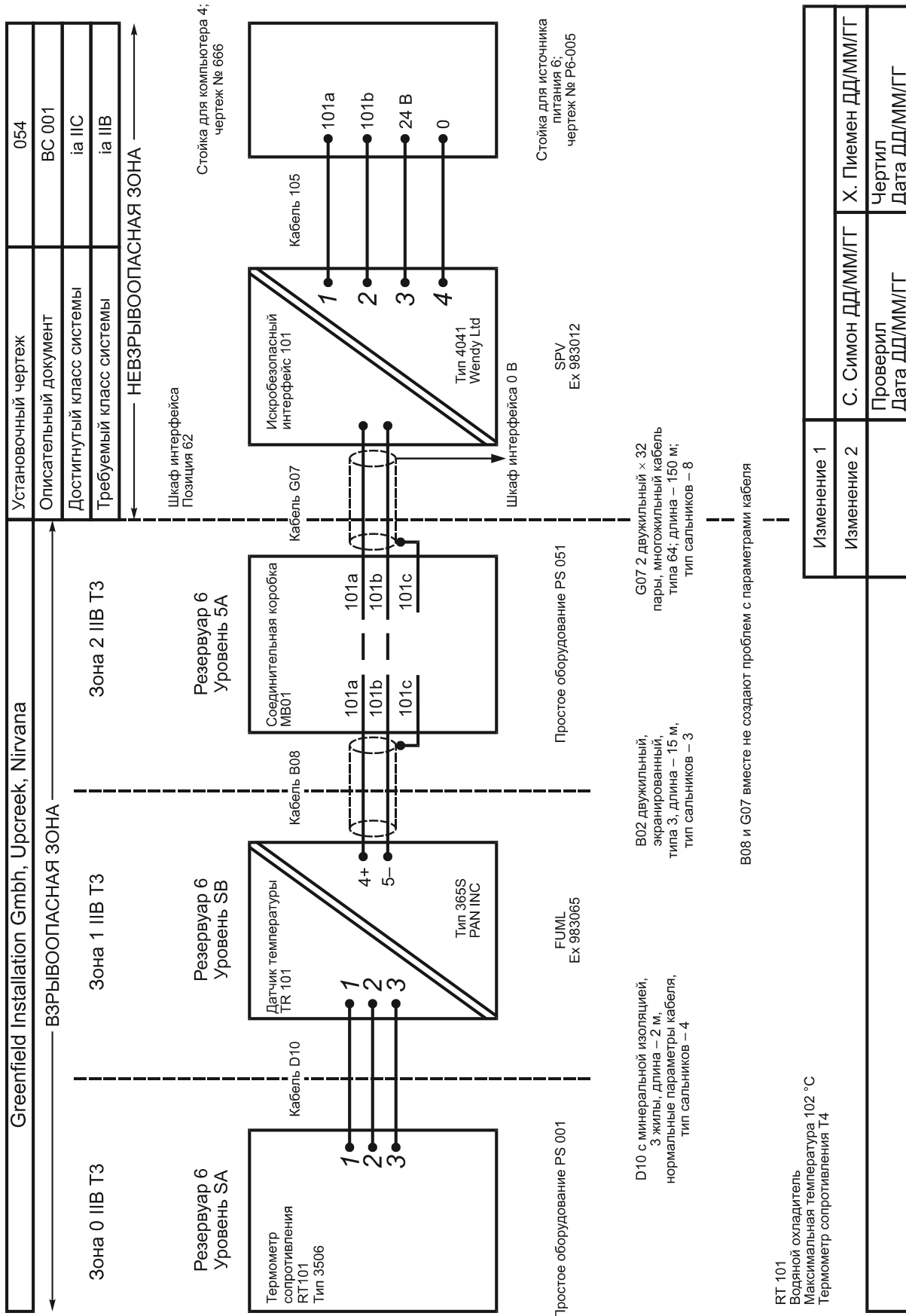
Рисунок Е.2 — Типовая схема соединений искробезопасной системы
