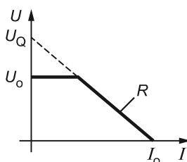
Рисунок С.1б — Трапециевидная характеристика
