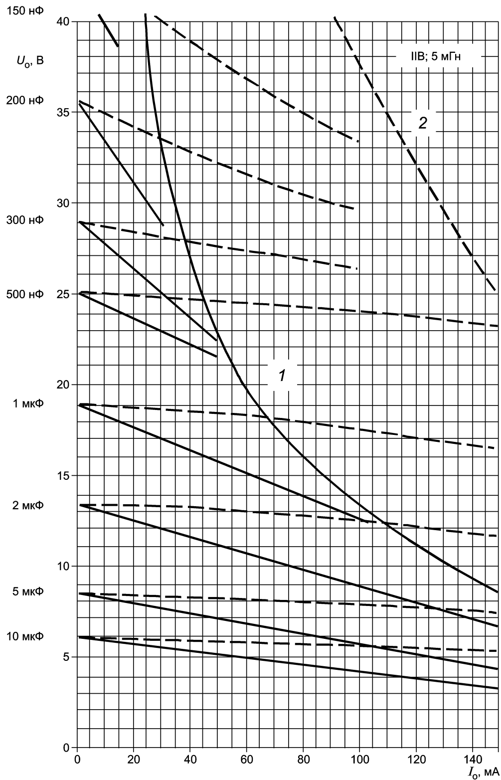
1 — максимальная индуктивность для источника с прямоугольной характеристикой; 2 — максимальная индуктивность для источника с линейной характеристикой
