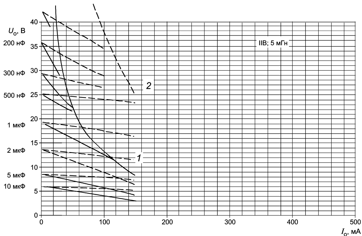
1 — максимальная индуктивность для источника с прямоугольной характеристикой; 2 — максимальная индуктивность для источника с линейной характеристикой
