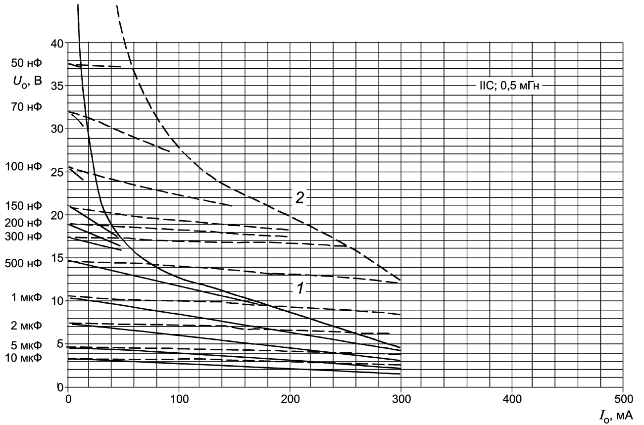
1 — максимальная индуктивность для источника с прямоугольной характеристикой; 2 — максимальная индуктивность для источника с линейной характеристикой
