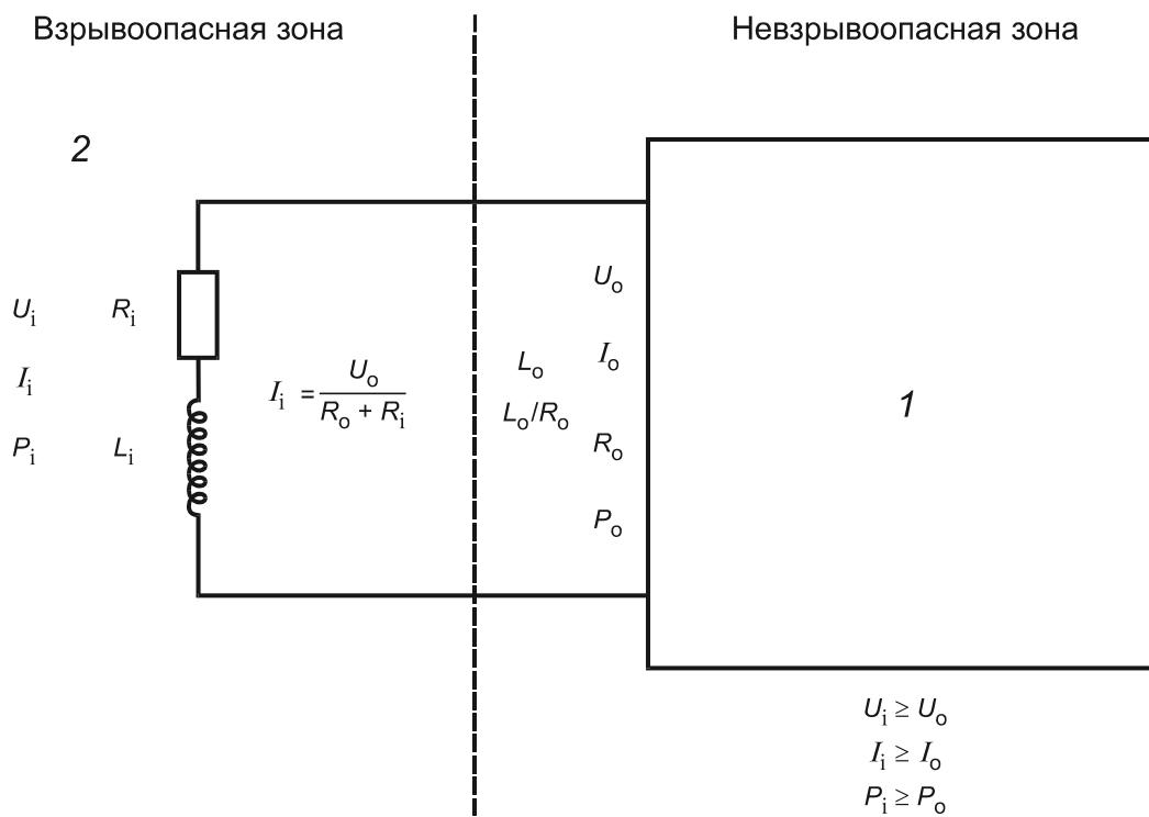
Рисунок D.1 — Типичная индуктивная цепь
