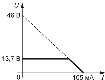
Рисунок С.3а — Выходные характеристики
