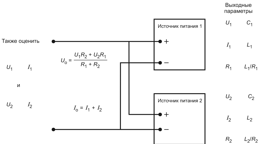
Рисунок В.2 — Источники питания, подключенные параллельно
