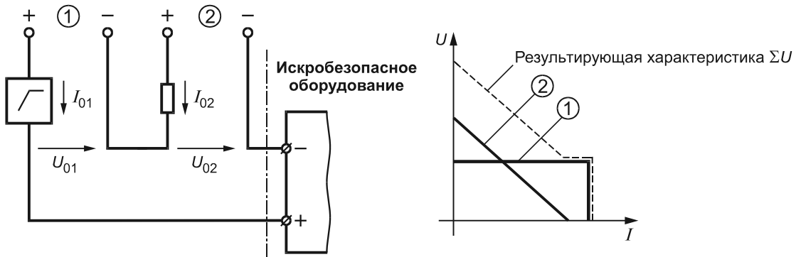
Рисунок С.2а — Последовательное подключение со сложением значений напряжения
