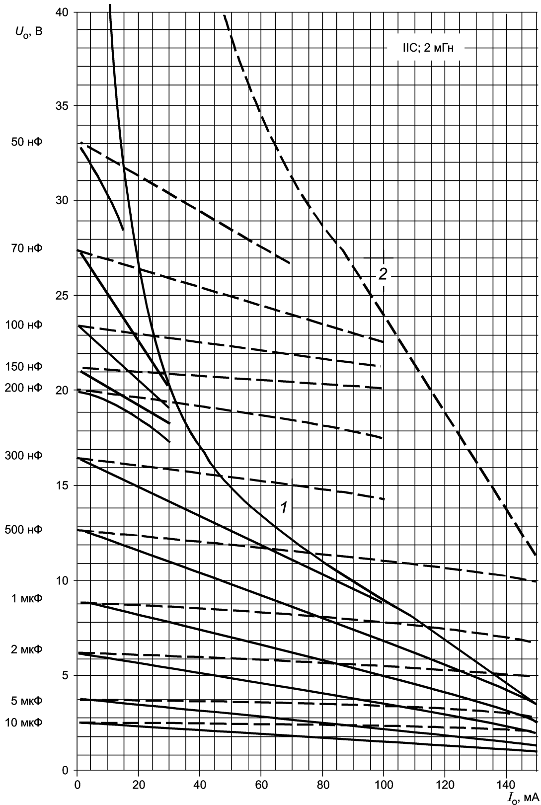
1 — максимальная индуктивность для источника с прямоугольной характеристикой; 2 — максимальная индуктивность для источника с линейной характеристикой
