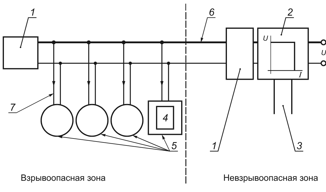
1 — оконечное устройство; 2 — источник питания; 3 — данные; 4 — ручной терминал; 5 — полевые устройства; 6 — магистральный кабель; 7 — ответвительный кабель
