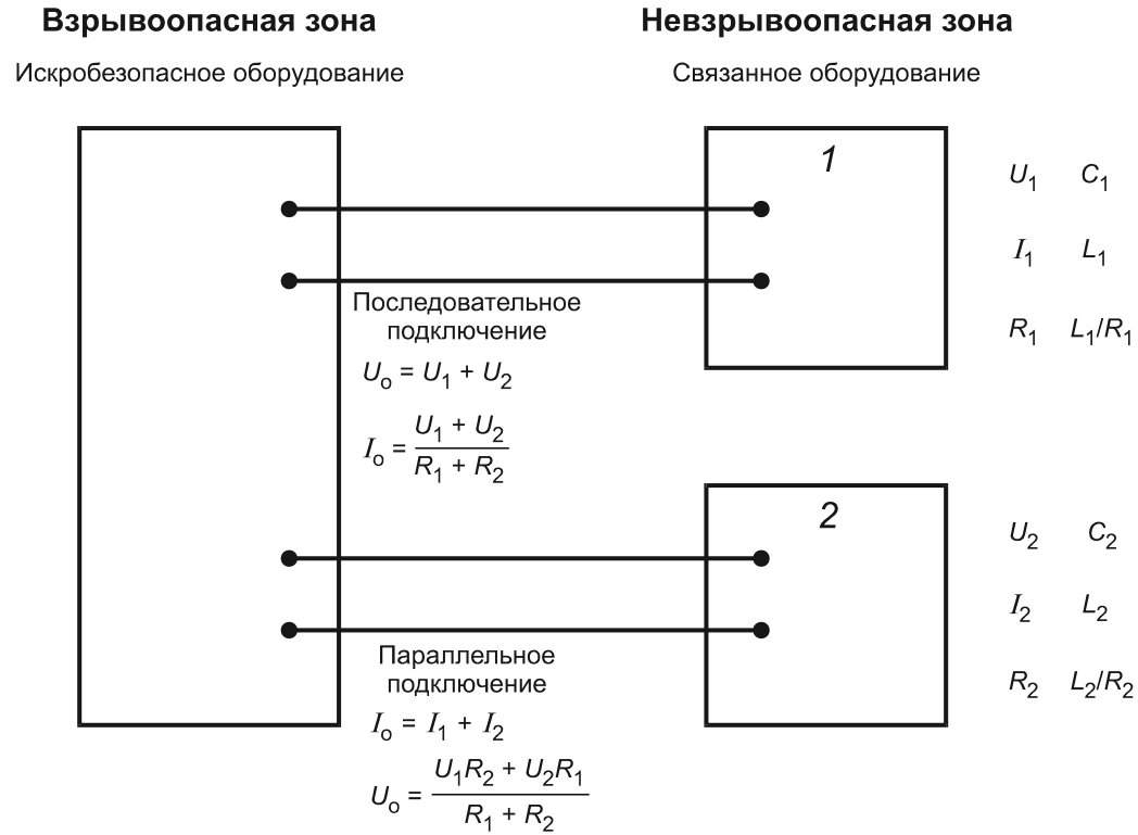
Рисунок В.3 — Произвольно подключенные источники питания
