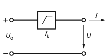
Рисунок С.1 — Характеристики эквивалентных цепей и выходов резистивных цепей
